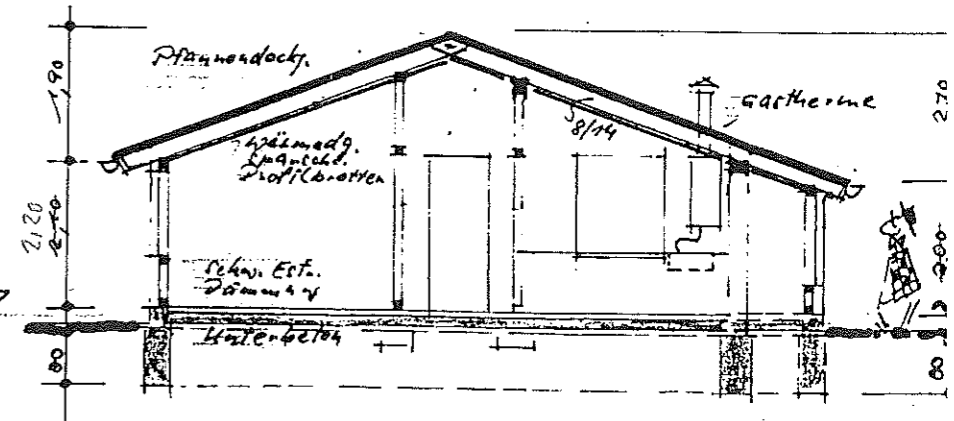
Querschnitt
