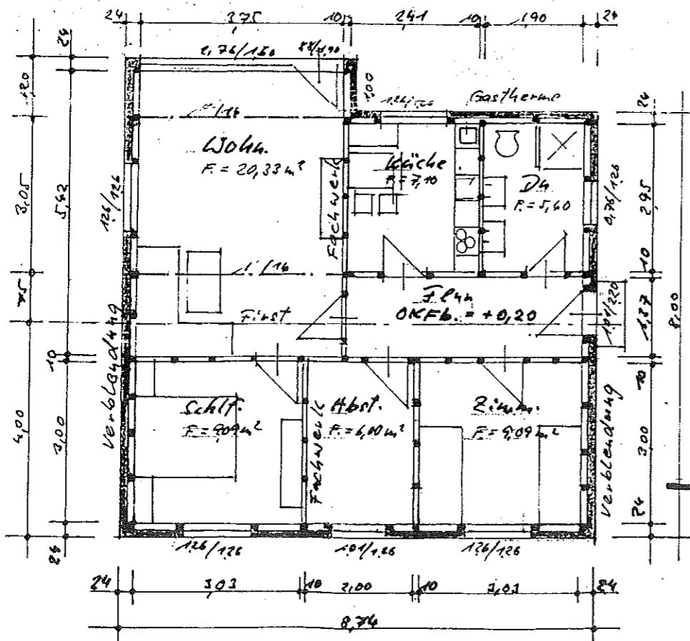
Grundriss
