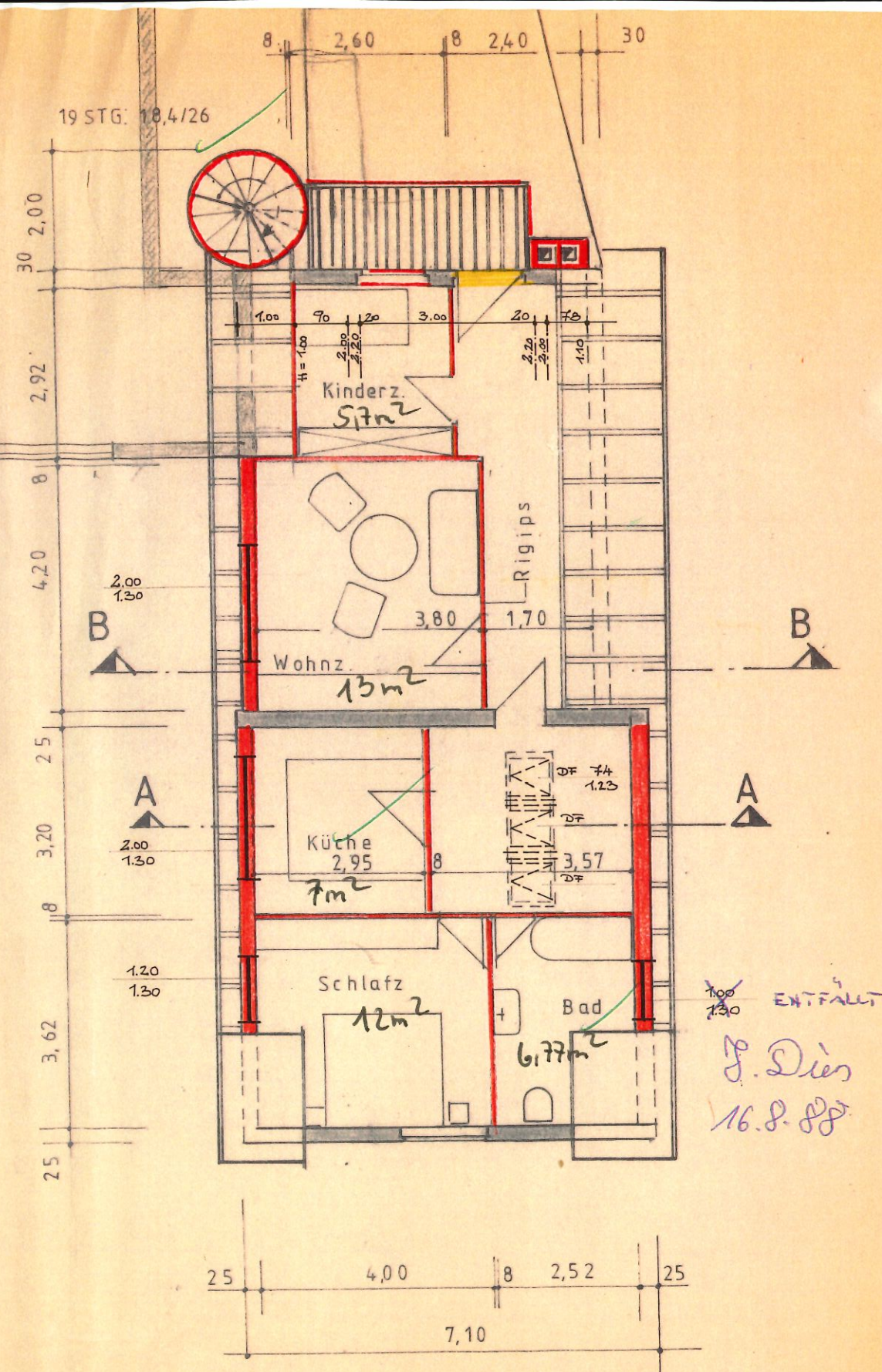
DACHGESCHOSS
